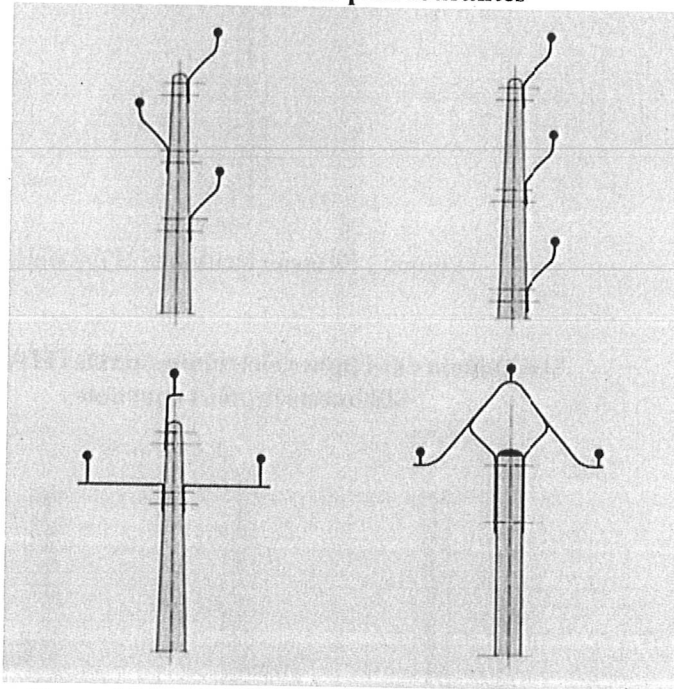
Figure 3 : Réseau électrique HTA - Technique rigide
